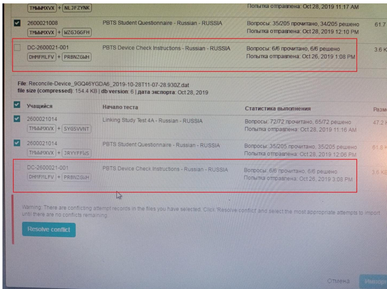
Рис.1. Конфликт при загрузке файлов с одним идентификатором.
